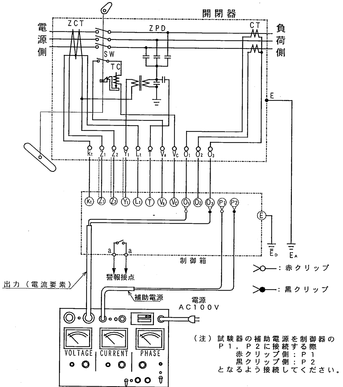
図11 SO試験動作回路
