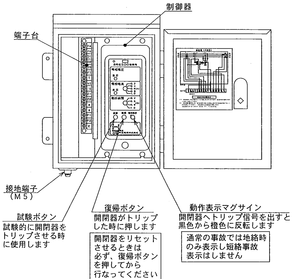
図4 各部の名称
