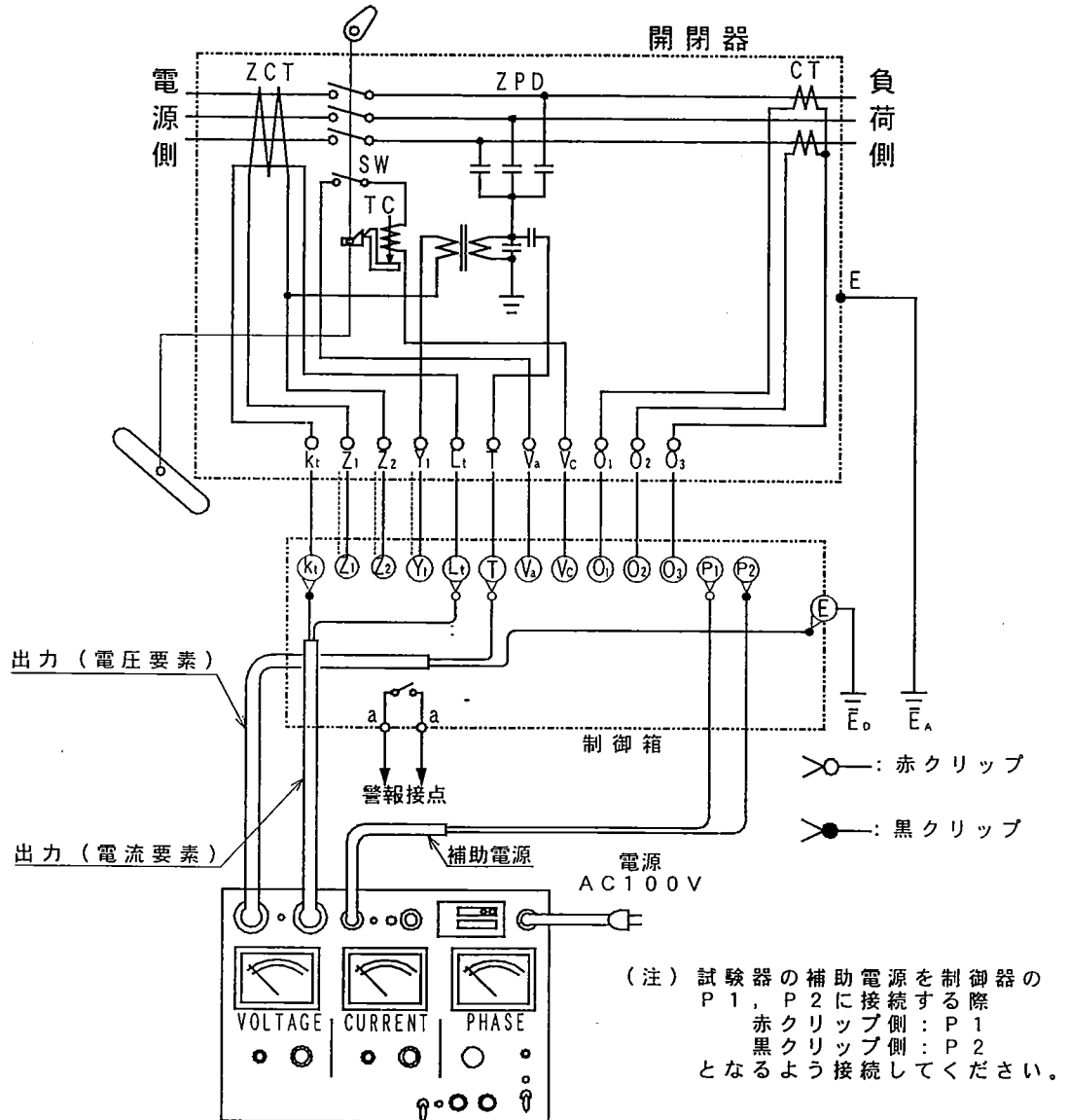
図10 地絡動作試験回路
