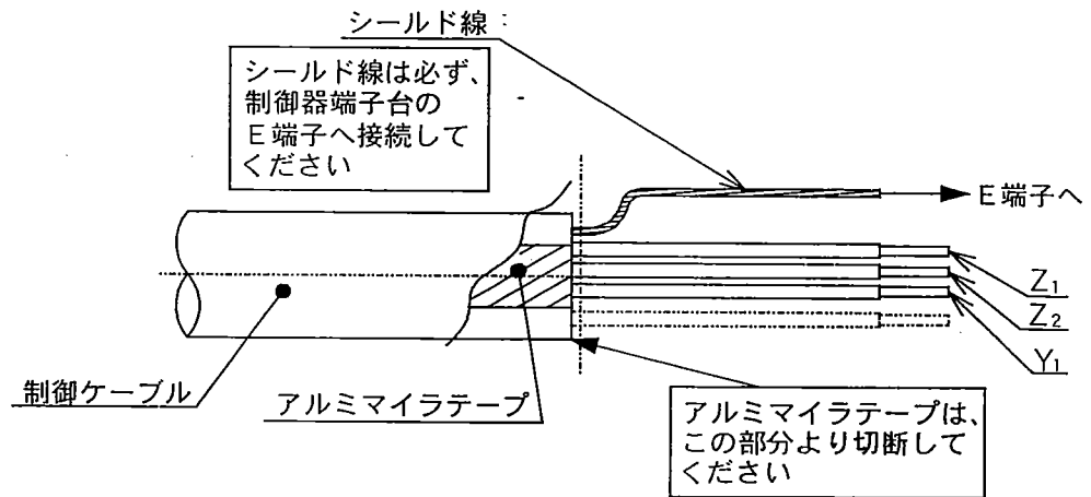
図7 シールド処理方法
