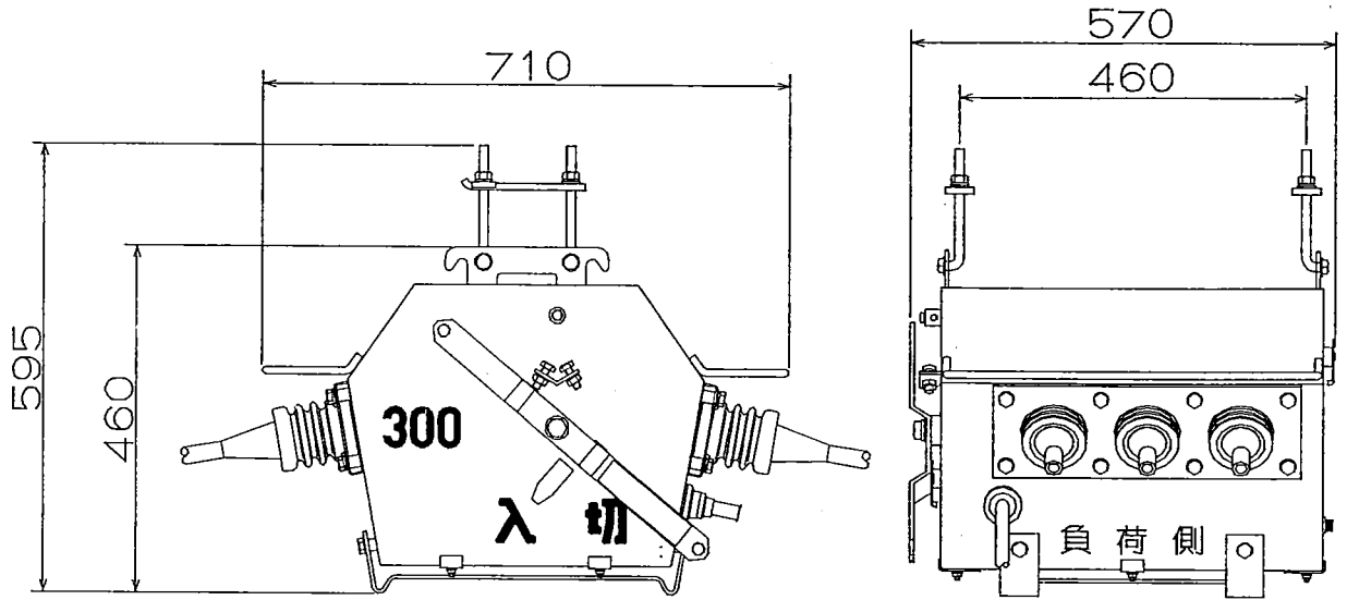
図1 外形寸法
