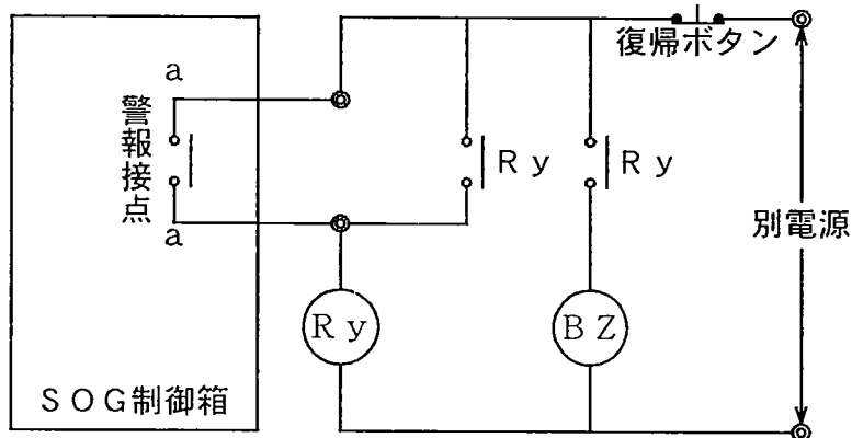
図12 警報回路例
