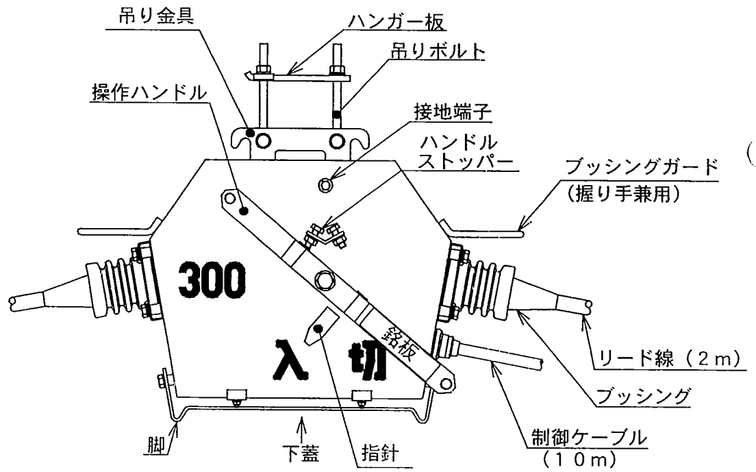
図2 各部の名称
