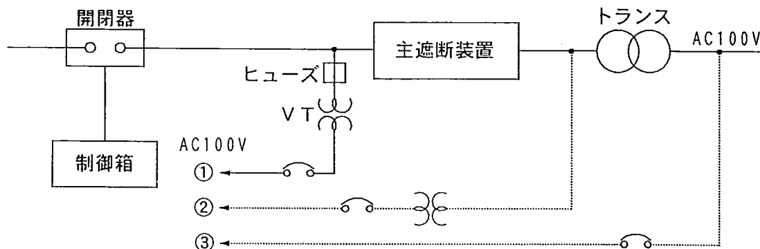
図9 制御電源のとりかた
