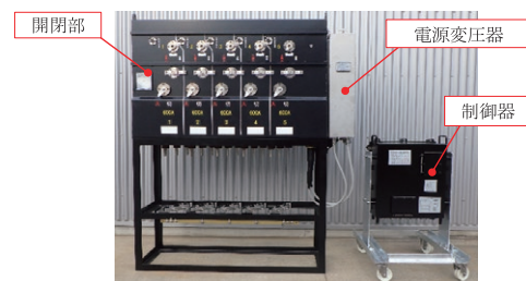
図1 製品外観
