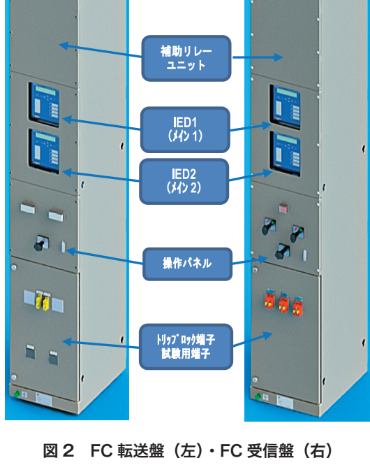
図 2 FC 転送盤（左）・FC 受信盤（右）
