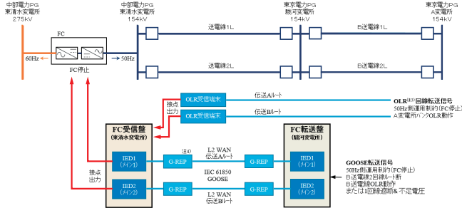
図 1 FC 転送盤・FC 受信盤のシステム構成
