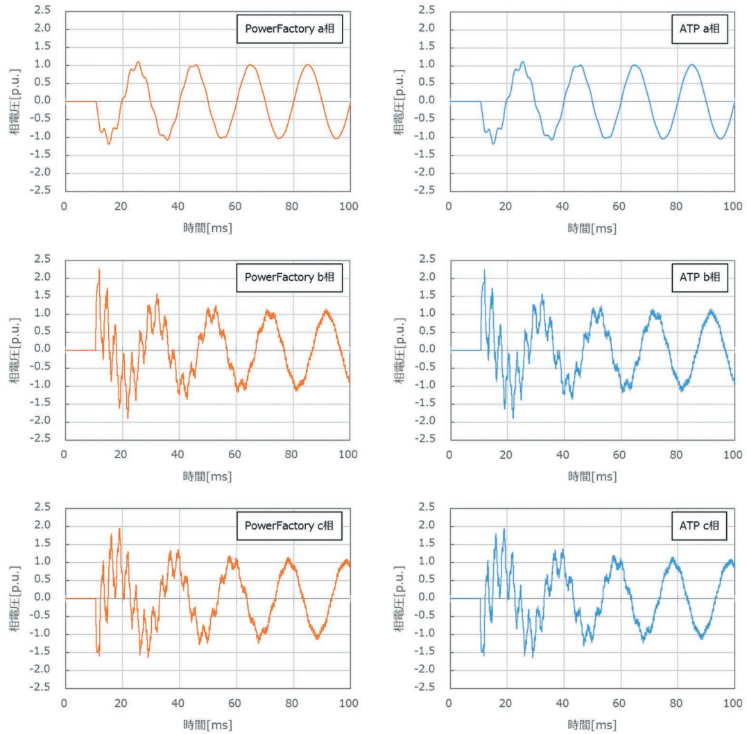
図4 投入サージ解析結果 (左: PowerFactory, 右: ATP)
