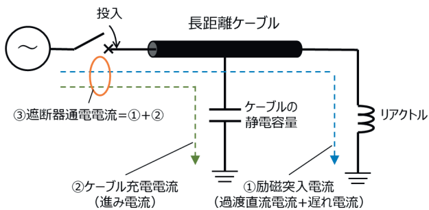
図1 電流零ミス現象の回路概略図
