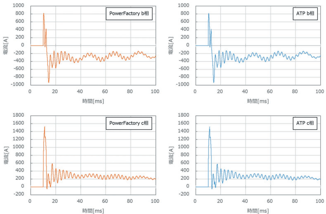
図5 電流零ミス解析結果 位相パターン1 (左: PowerFactory, 右: ATP)
