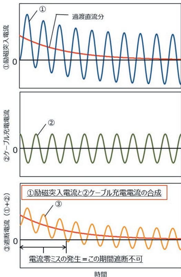
図2 電流零ミス現象波形イメージ
