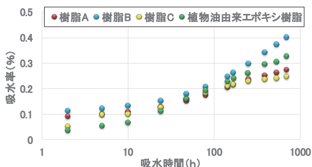
図5 各樹脂の吸水時間と吸水率の関係
