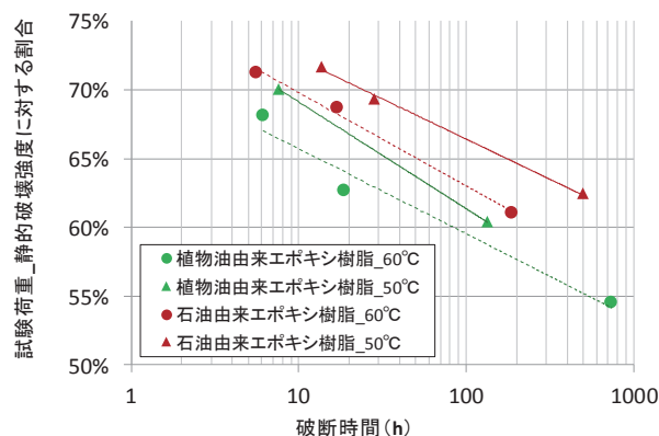
図 4 クリープ特性比較 (平均値)
