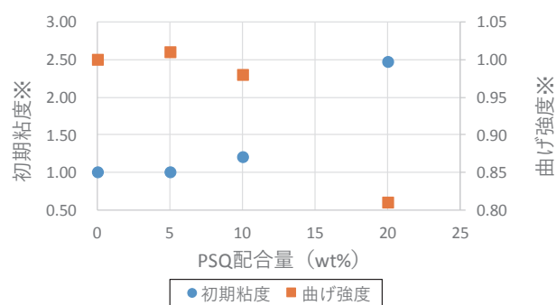
図2 初期粘度および曲げ強度とPSQ配合量の関係
