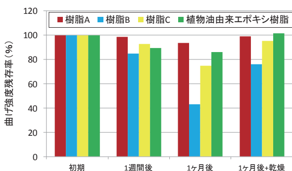
図6 各樹脂の吸水時の曲げ強度残存率
