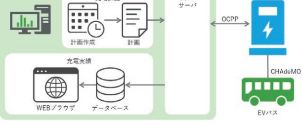
図1 運行管理と一体化したEMS (2)
